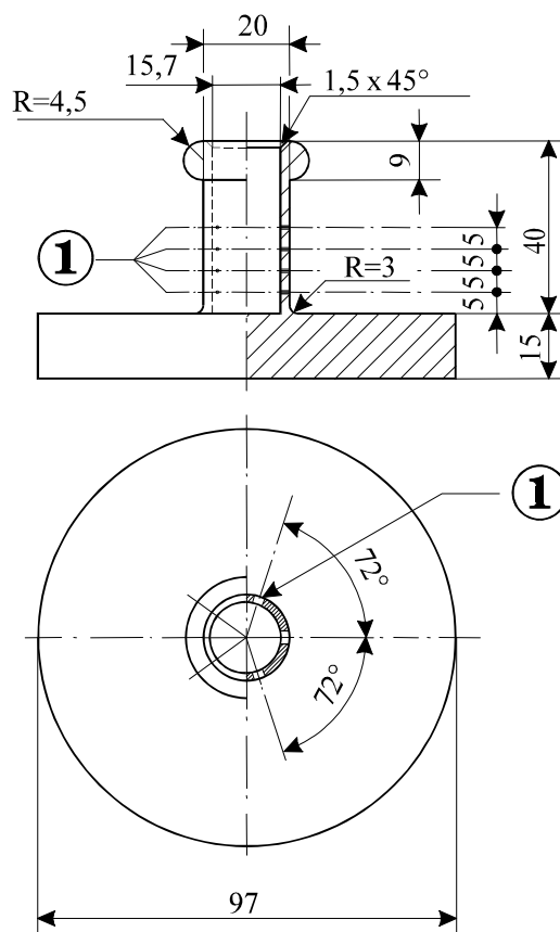
Abb. 3: Hohlbronzezyylinder, einseitig verschlossen Aufriss und Grundriss; Maße in mm
